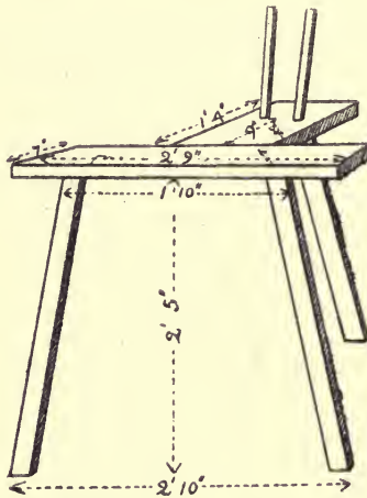
Fig. 5. Basket-loading Stand or Chargeur.
